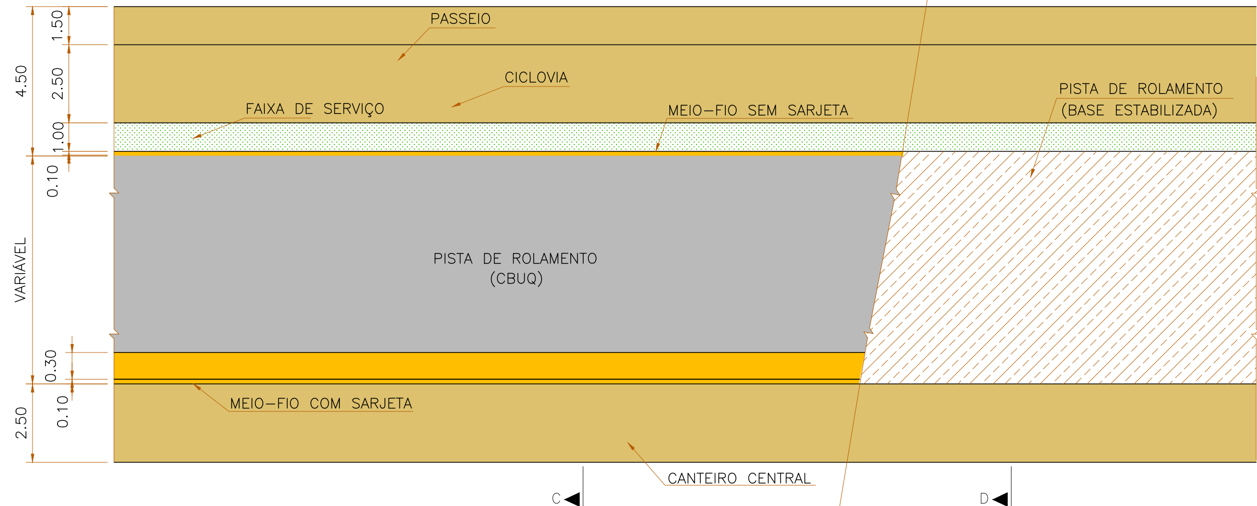
PAVIMENTAÇÃO TÍPICA – 02 PLANTA ESC. 1:100
