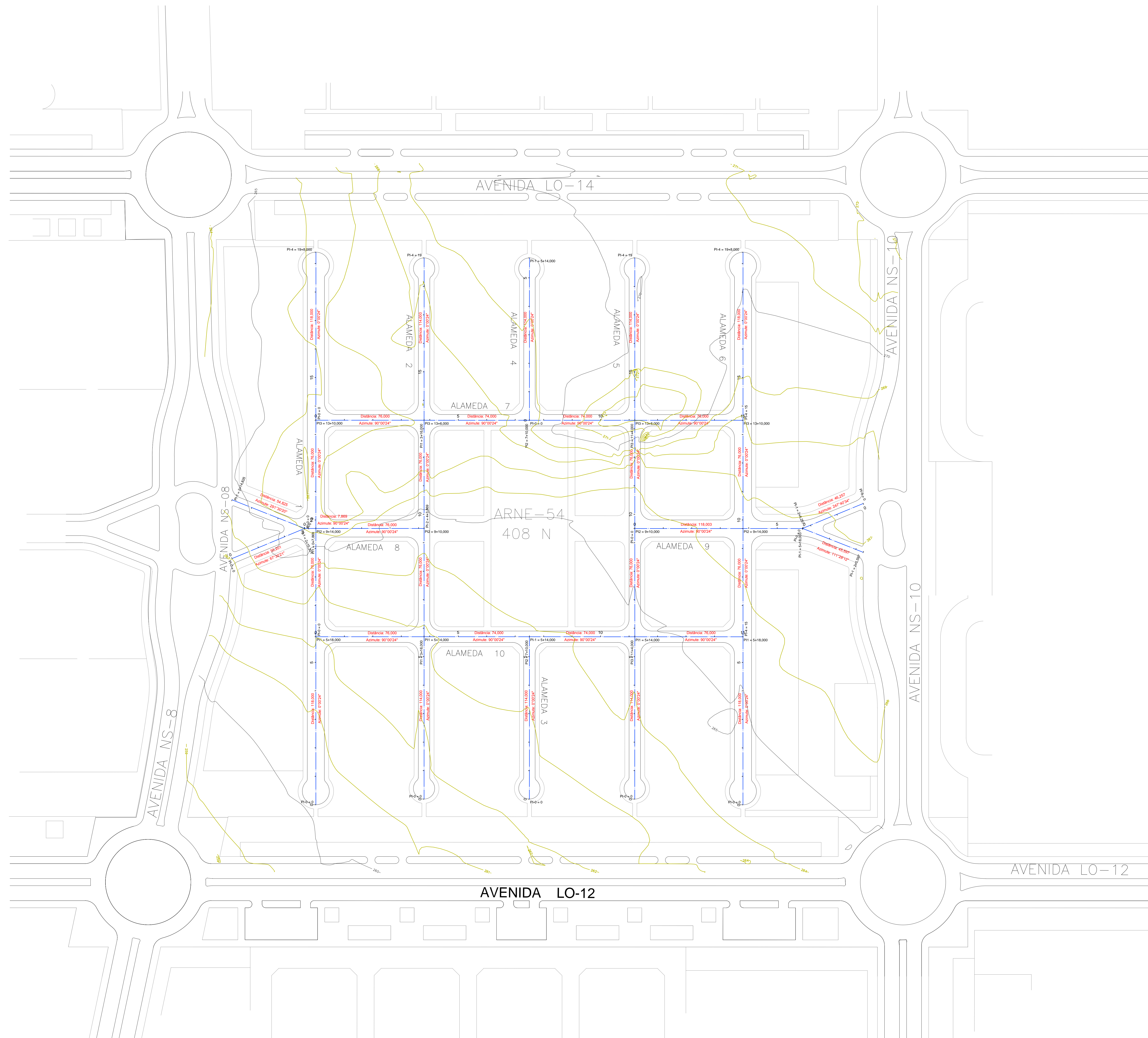
Planta de Terraplanagem Escala: 1 / 1.000
